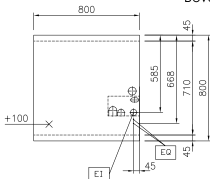
Boven aanzicht
