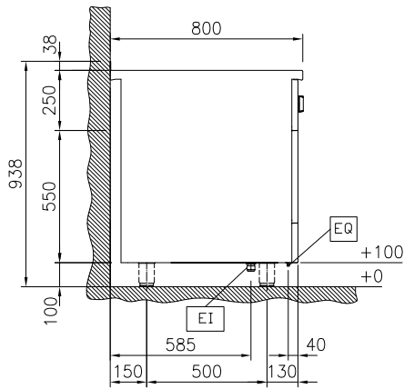
Zij aanzicht
